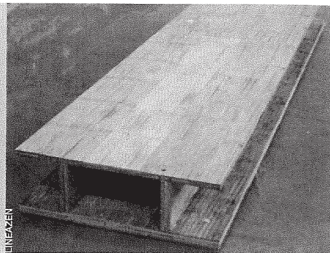
Le système de construction bois original mis au point par Lineazen.
